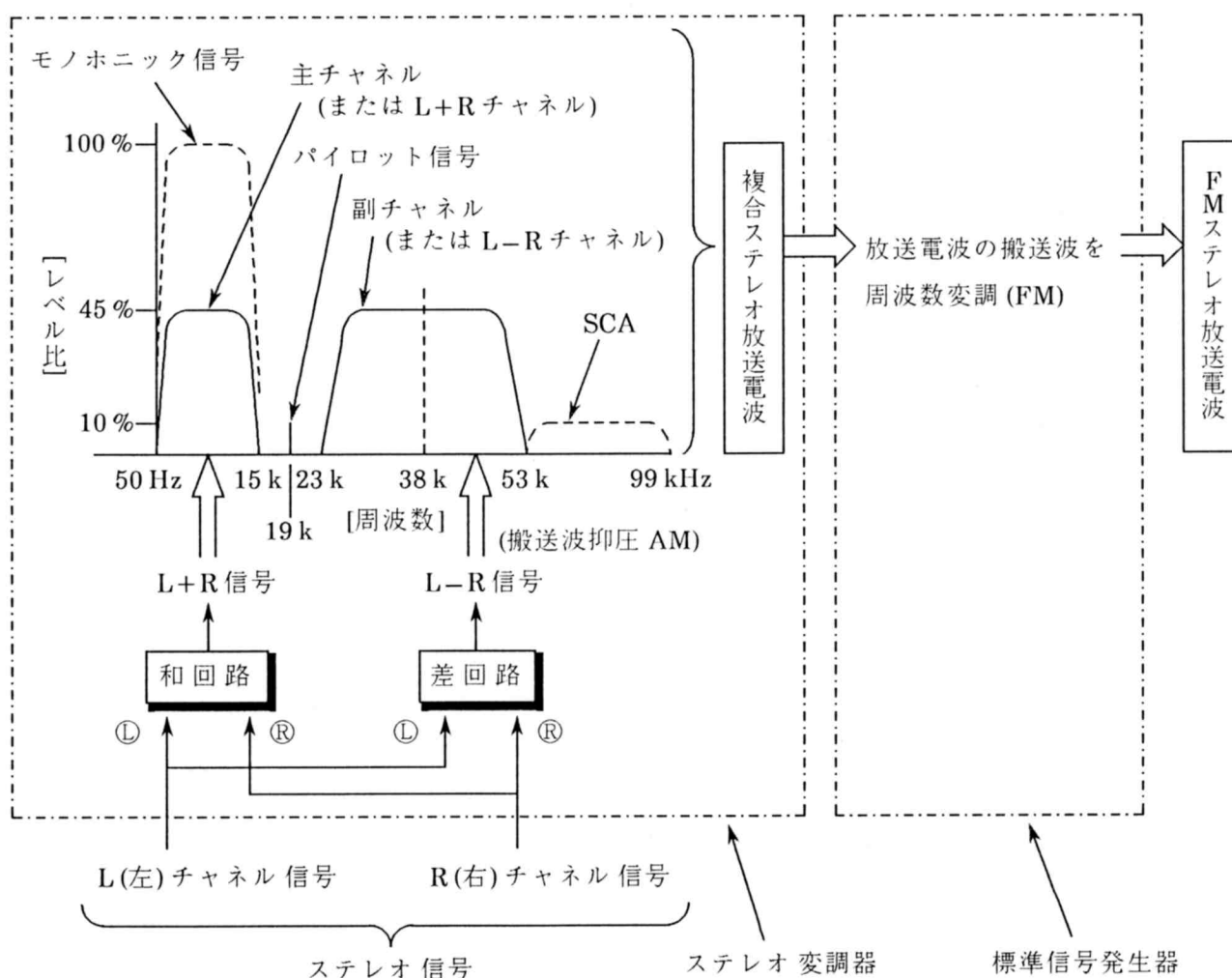
1-2図 FMステレオ放送の概要
