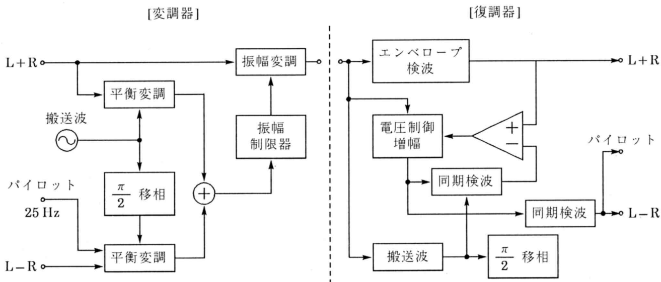
1-4図 C-QUAM方式
