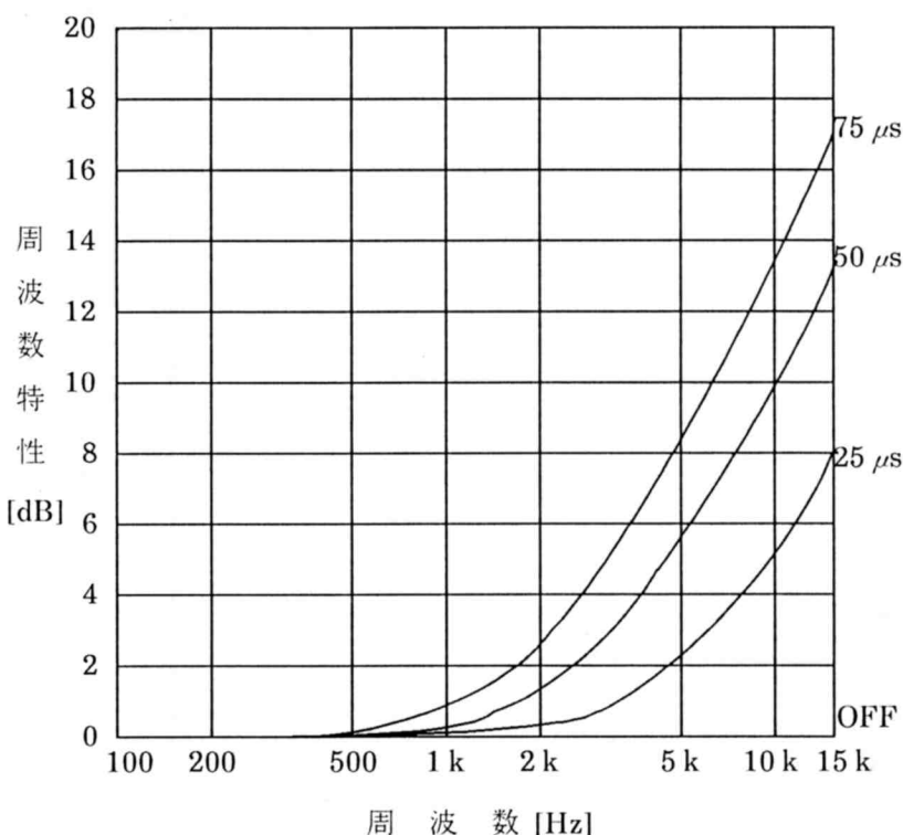
4-2図 標準プリエンファシス特性
