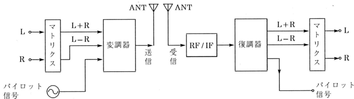
1-3図 AMステレオの基本ブロック図
