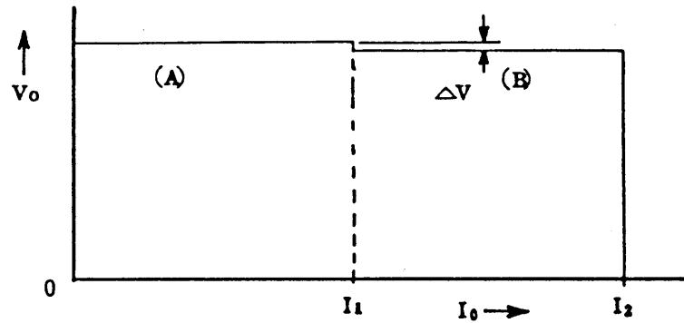
第 3 - 7 図 特 性 図
