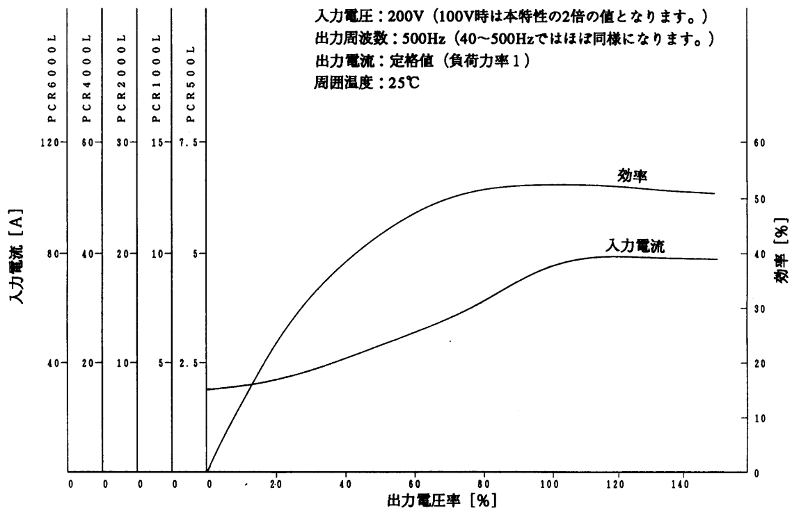
出力電圧—入力電流、効率特性 ACモード [標準値]
