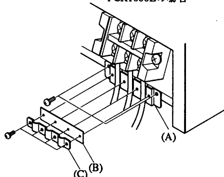
PCR4000L, 6000Lの場合
