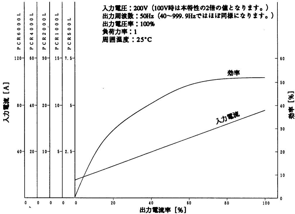
出力電流—入力電流、効率特性 ACモード [標準値]
