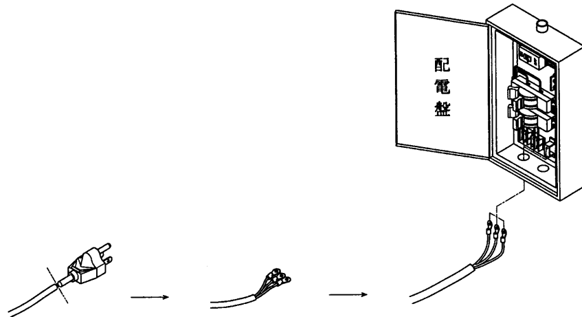
200V系の場合（配電盤への接続）
