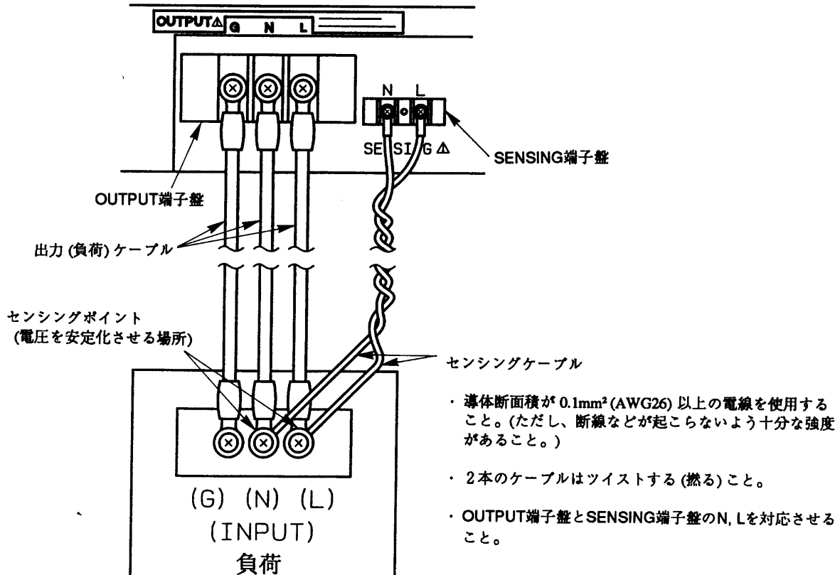
センシング端子盤の結線方法
