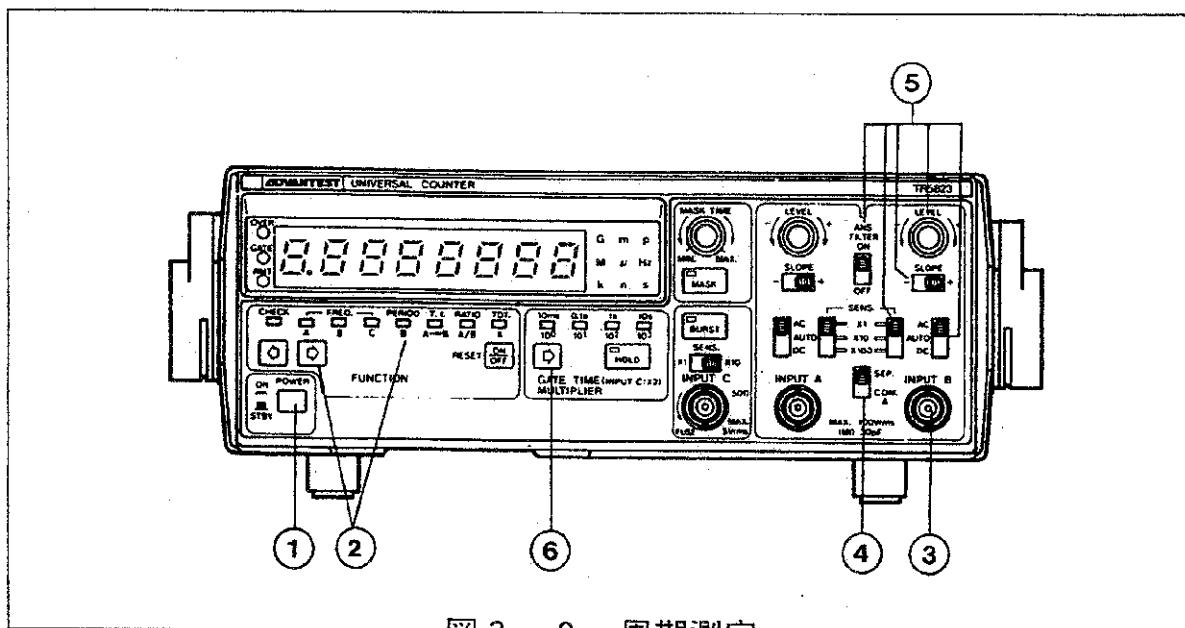
図 3-9 周期測定
