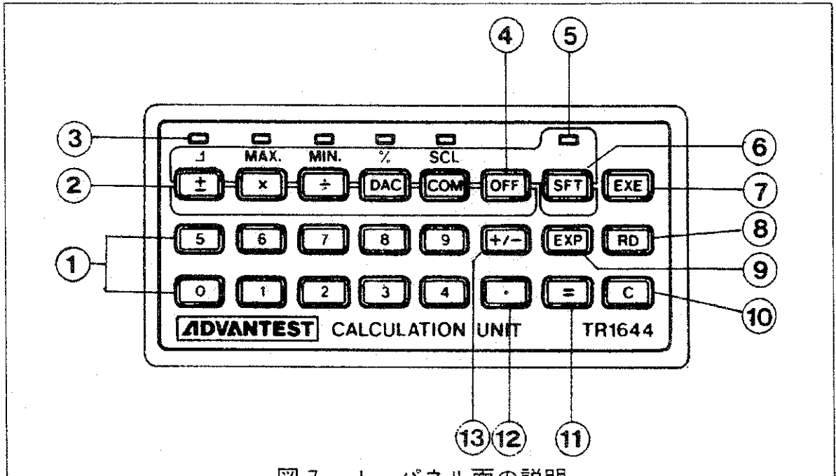
図 7-1 パネル面の説明
