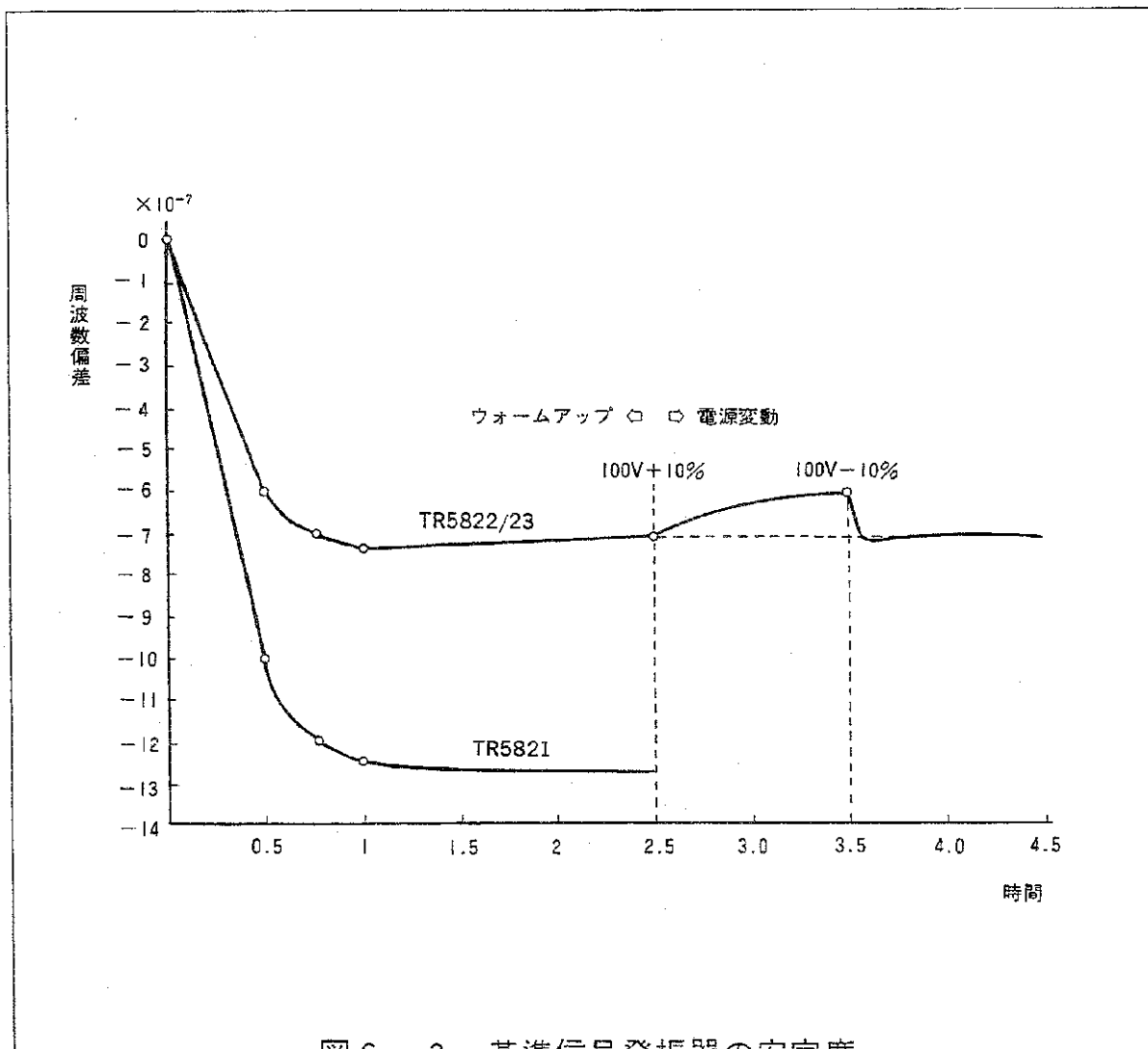
図 6 - 2 基準信号発振器の安定度
