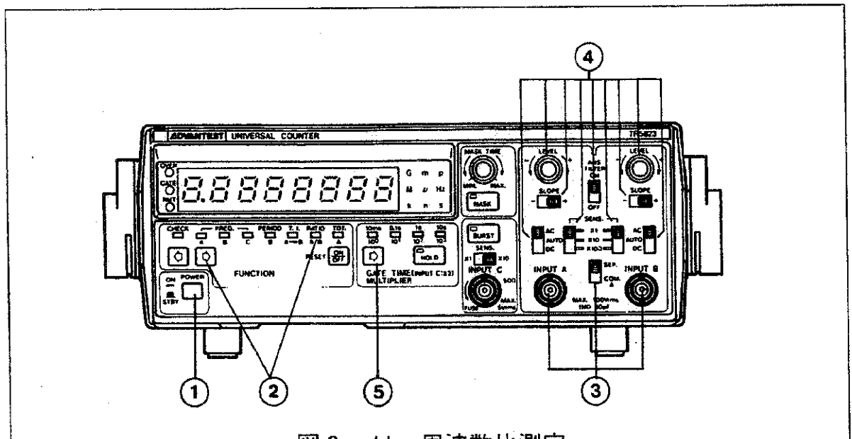
図 3-11 周波数比測定
