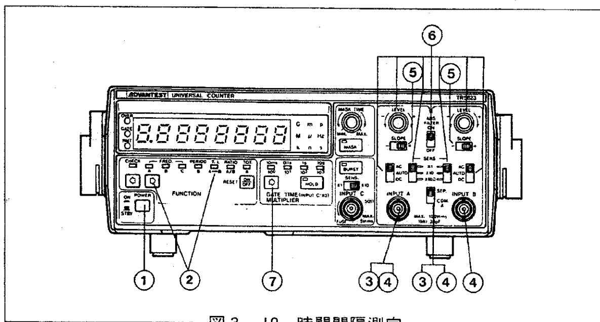
図 3-10 時間間隔測定
