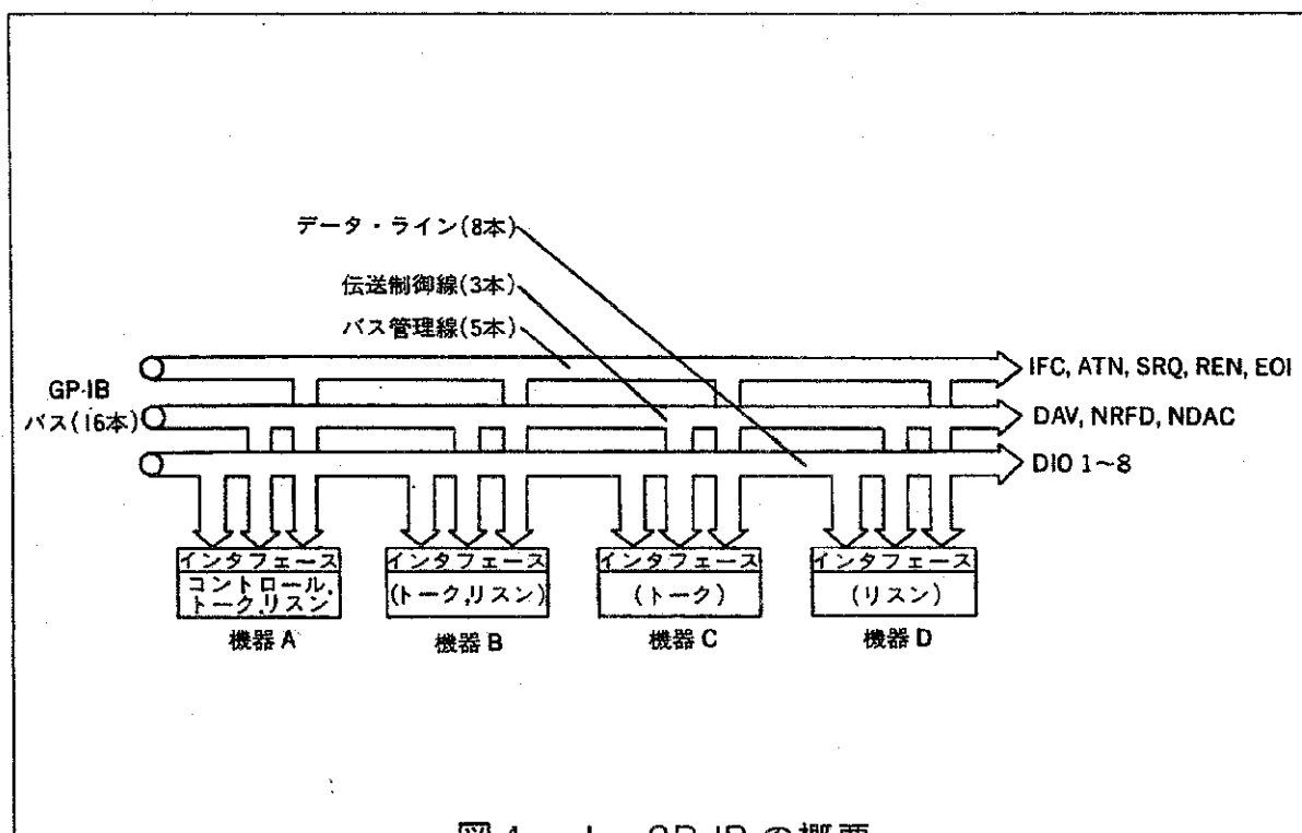
図 4 - 1 GP-IB の概要
