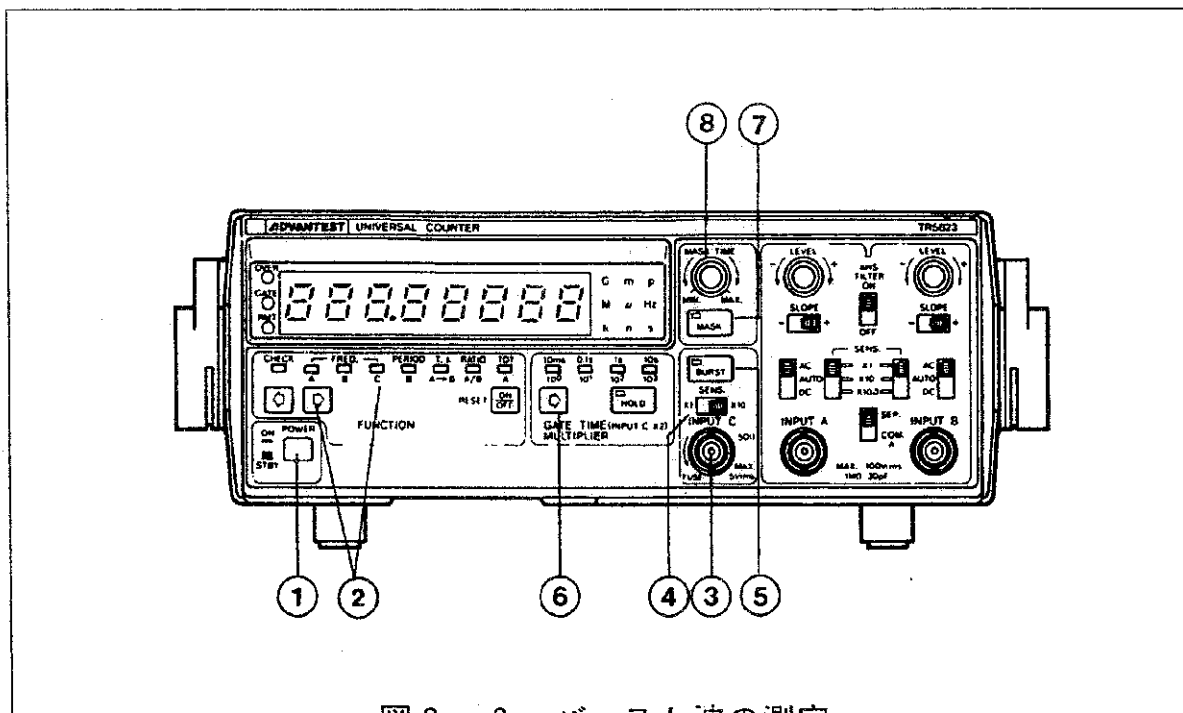
図 3 - 8 バースト波の測定
