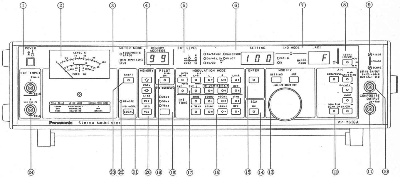
正面图
