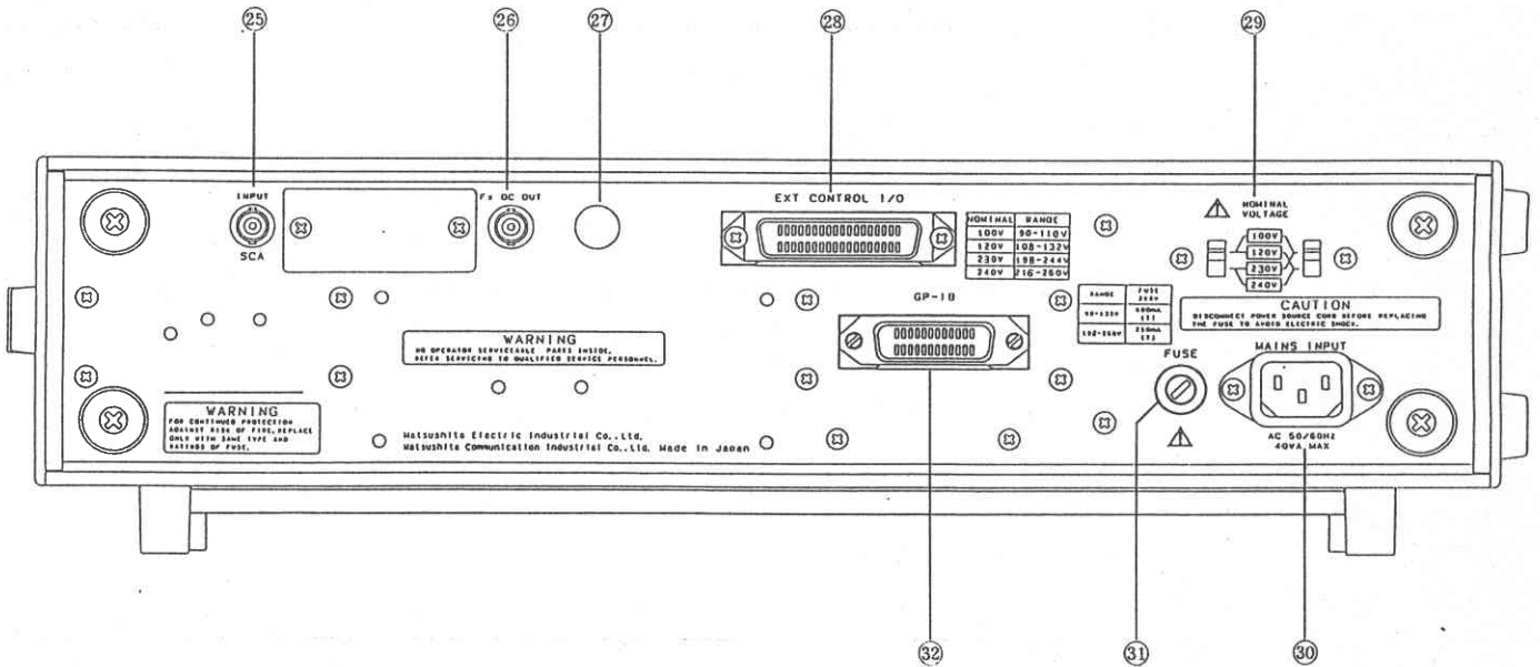
背面图
