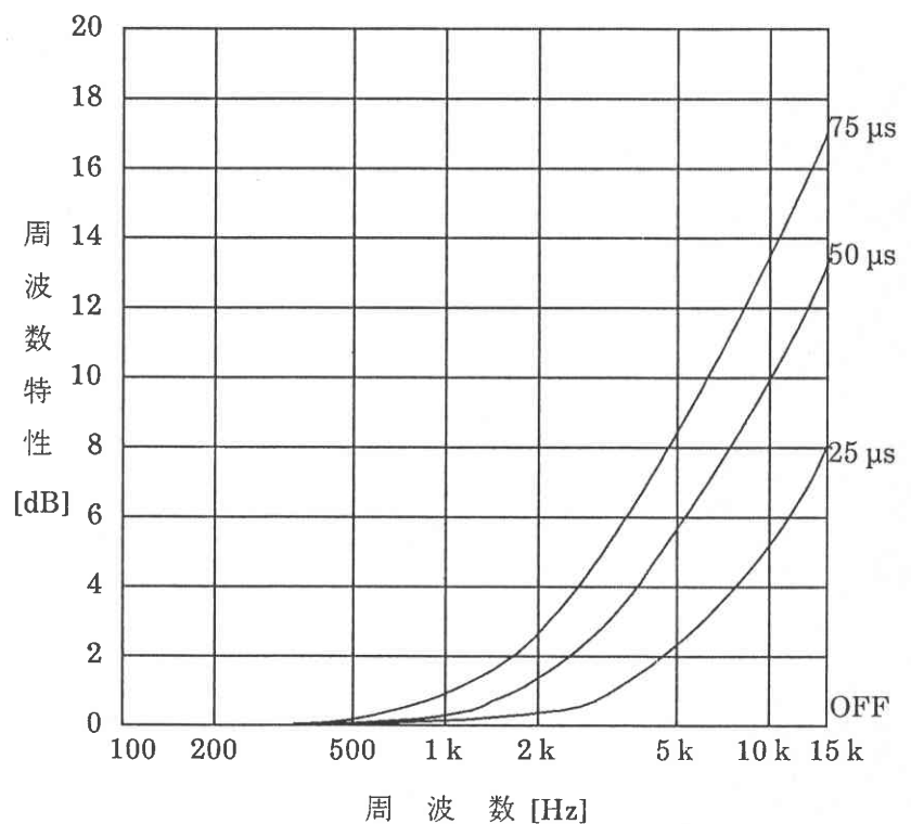
4-1図 標準プリエンファシス特性
