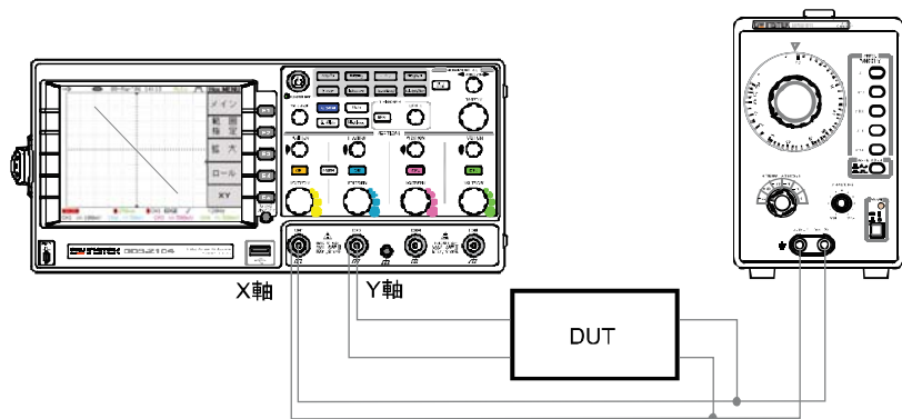
図 5 位相特性の測定
