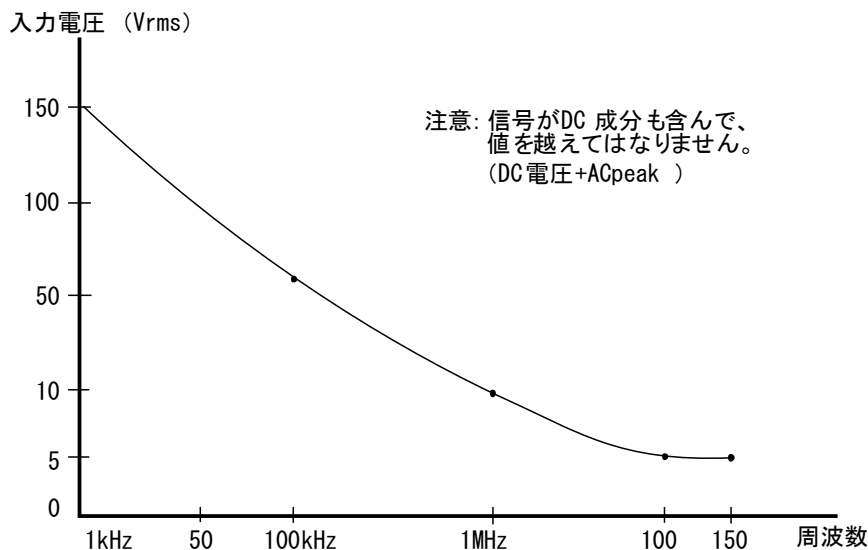
図6 最大入力電圧対周波数
