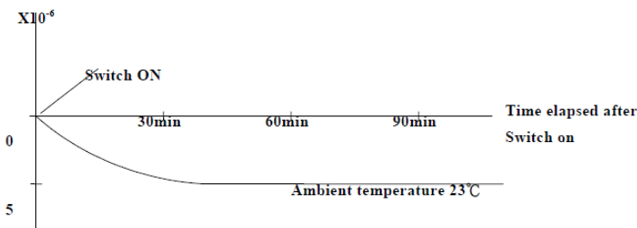
図9 水晶発振子の電源投入後の変化特性
