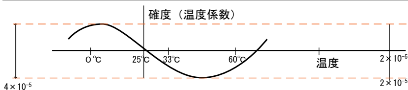
図8 水晶発振子の温度特性
