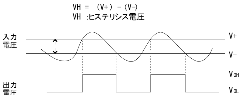
図2 シュミット回路の動作
