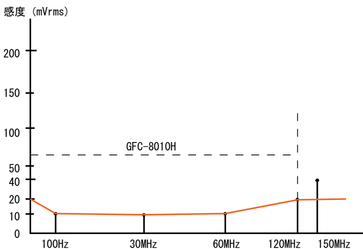
図5 入力感度特性
