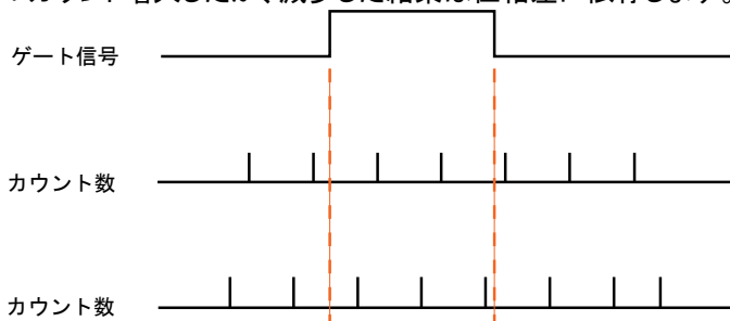
図 7 \pm 1 カウントエラー
