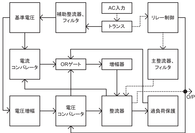
ブロック図
